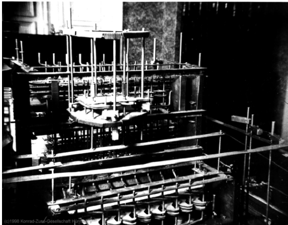
Speicher der Z1 (ca. 1937).
