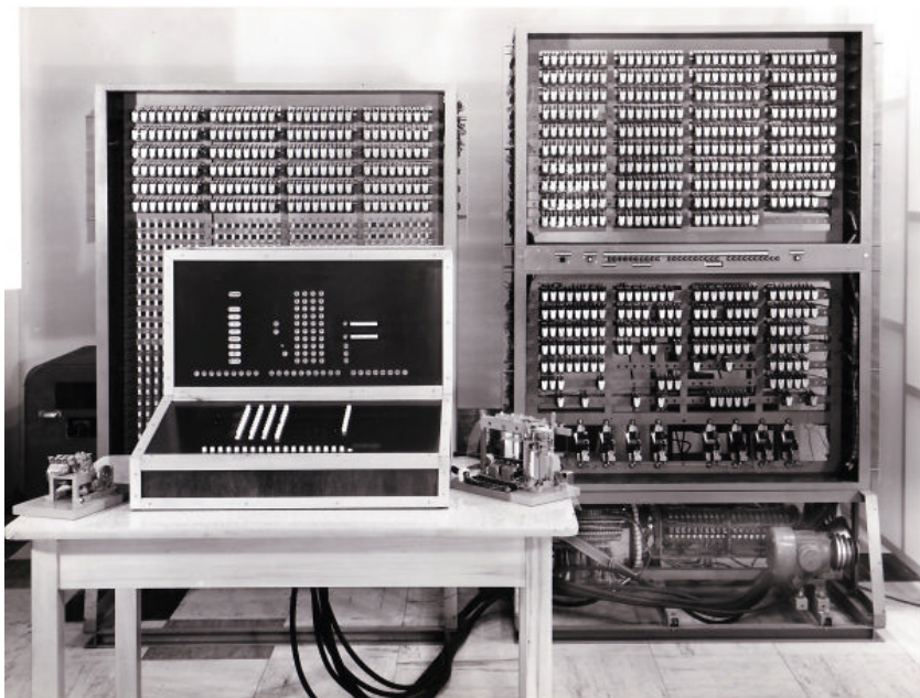
Nachbau der Z3 (1961).
