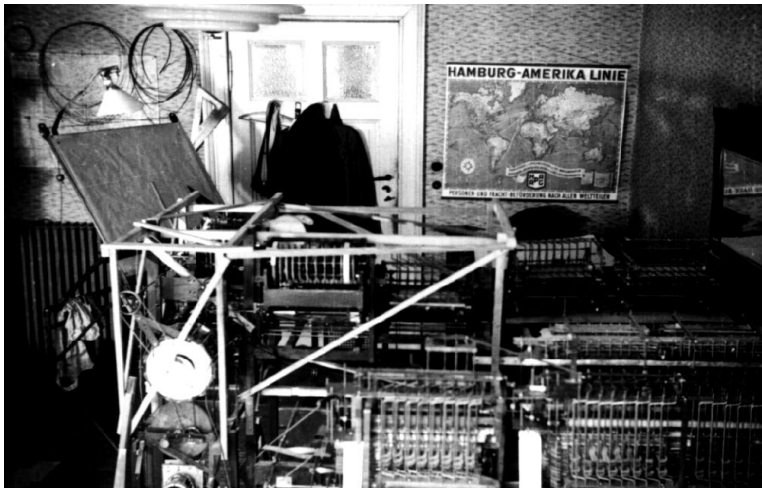
Speicher der Z1 (ca. 1937).
